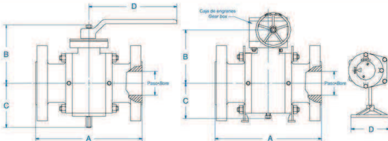
Dimensiones • Dimensions
