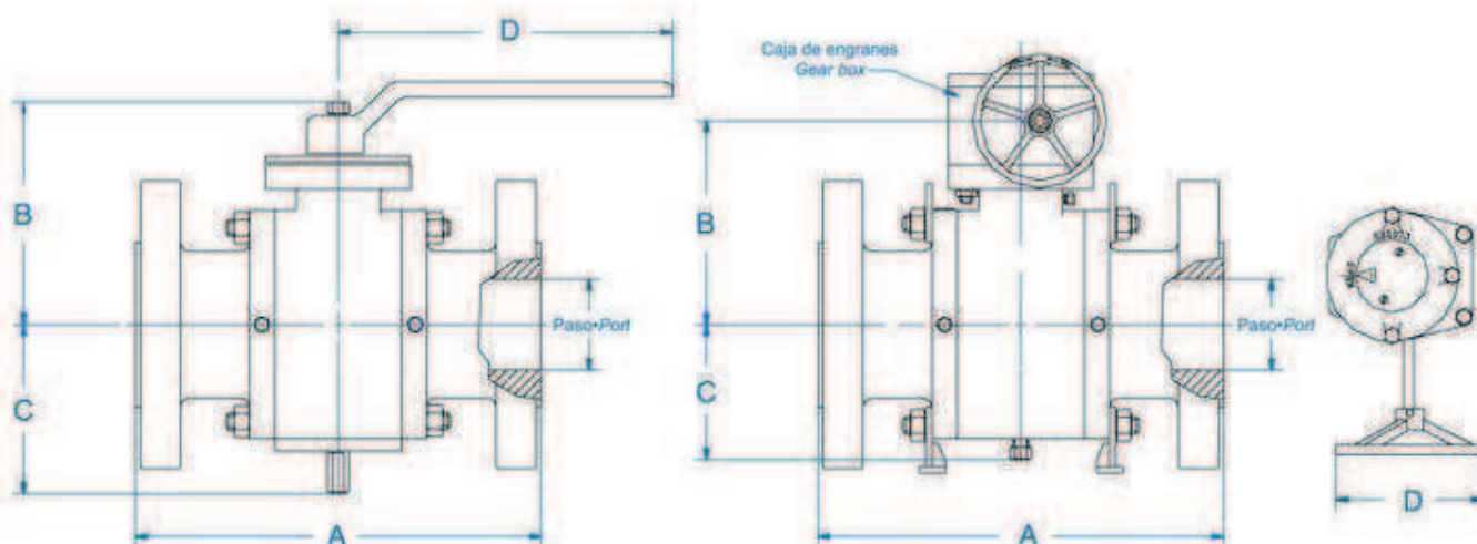
Dimensiones • Dimensions
