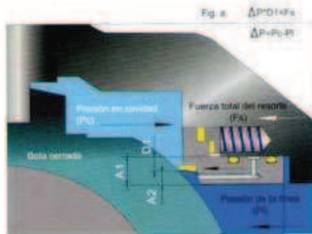
Fig. a \Delta P \cdot D1 < F_s \Delta P = P_c - P_l Cuando la presión de la cavidad ( P_c ) es más baja que el resorte del asiento y la presión de la línea ( P_l ), i.e.
