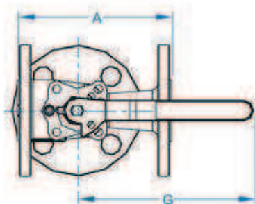
Dimensiones • Dimensions
